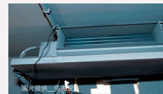
裝設在天花板下的VAV室內送風機，可依溫度來自動開啟或關閉送風。
